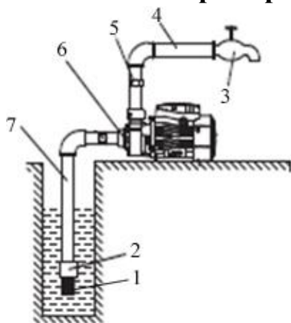
Правильная установка насоса.
